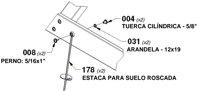
DETALLE - A
