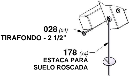
DETALLE - B
