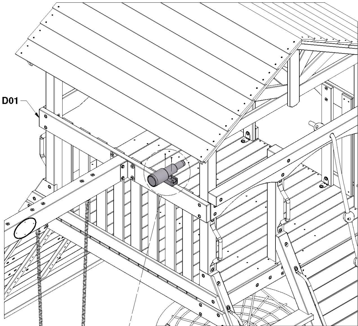
086 (x2) TORNILLO - 1 1/2"
